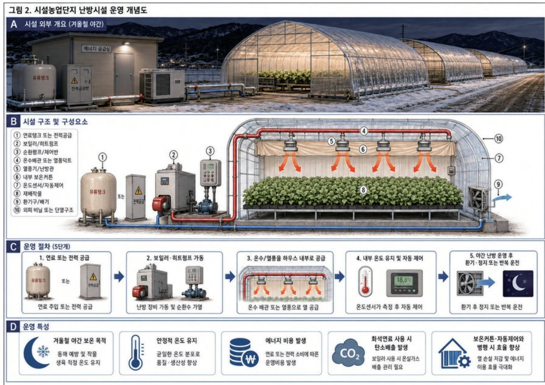
그림 2. 시설농업 단지의 난방시설 운영 개념도.
