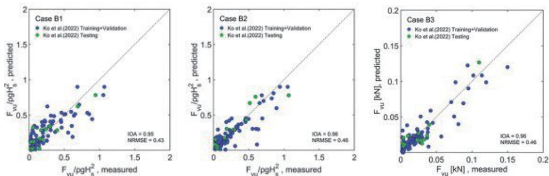
그림 5. Ko et al.(2022)의 자료로 구축한 인공신경망 모델(B1~B3)의 F_{vu} 예측값과 예측값 비교
