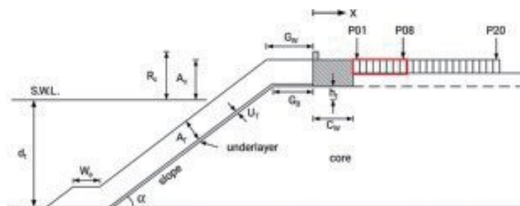
그림 2. Lee et al.(2022)의 실험 단면 및 매개변수 정의
