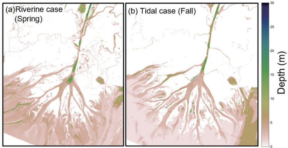
그림 2. AVIRIS-NG로 추정된 Wax Lake Delta의 수심 분포: (a) 2021년 봄, (b) 2021년 가을(Kwon et al., 2024, 2025).
