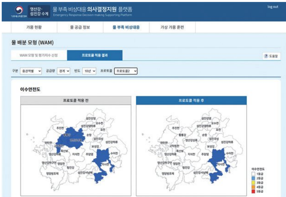
그림 4. WAM을 이용한 대응 전·후 물 부족 규모 비교
