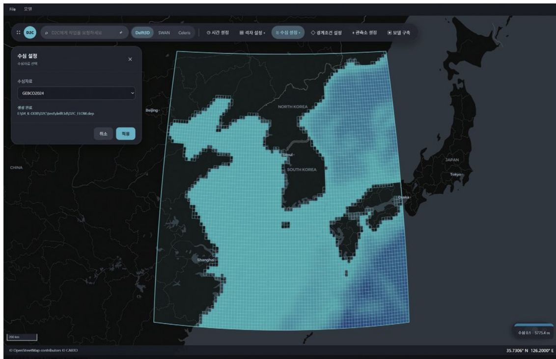
그림 2. Delft3D FLOW 탭에서 격자·수심·개방경계를 적용한 화면
