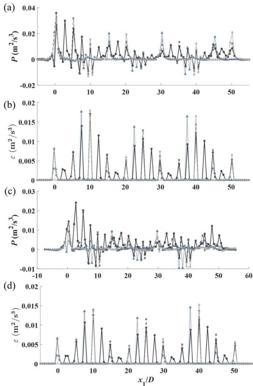
그림 3. 실린더 배열에 따른 난류 특성의 흐름방향 분포: (a) Type A의 난류 생성률, (b) Type A의 난류 소산률, (c) Type B의 난류 생성률, (d) Type B의 난류 소산률; 원(○) A1/B1, 사각형(□) A2/B2, 삼각형(△) A3/B3, 마름모(◇) A4/B4.
