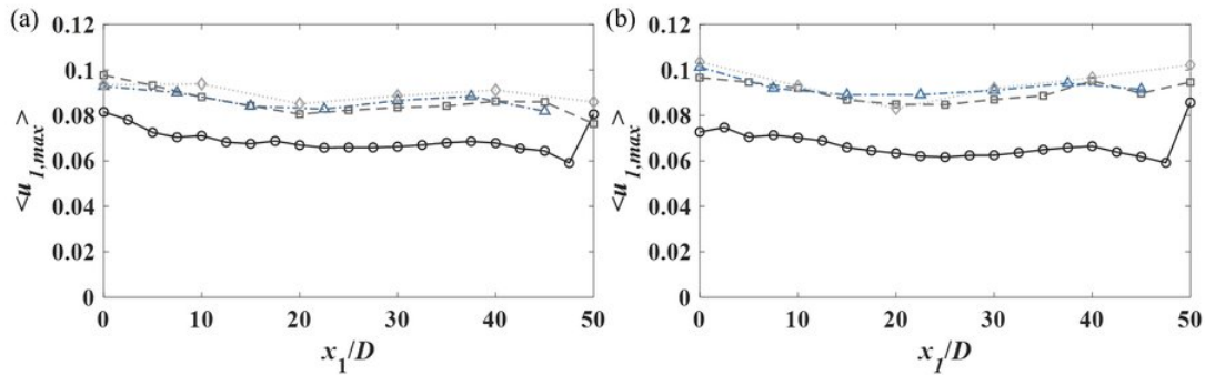
그림 2. 실린더 중심에서 1D 하류 지점에서의 배열 내부 최대 위상평균 흐름방향 유속 분포: (a) Type A와 (b) Type B; 원(○) A1/B1, 사각형(□) A2/B2, 삼각형(△) A3/B3, 마름모(◇) A4/B4.
