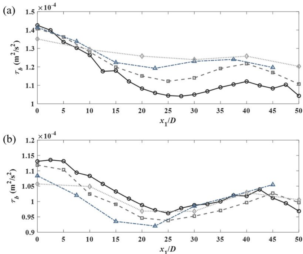
그림 4. 실린더 배열 내부 최대 위상평균 바닥전단응력의 흐름방향 분포: (a) Type A와 (b) Type B; 원 (○) A1/B1, 사각형(□) A2/B2, 삼각형(△) A3/B3, 마름모(◇) A4/B4.
