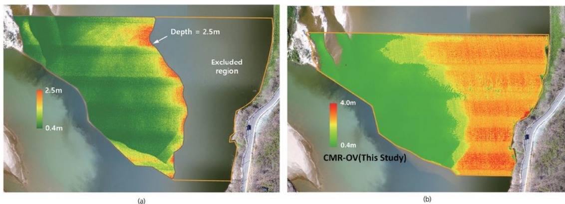
그림 4. 낙동강 본류의 초분광 수심도 비교: (a) OBRA, (b) CMR-OV(김도현 등, 2026).
