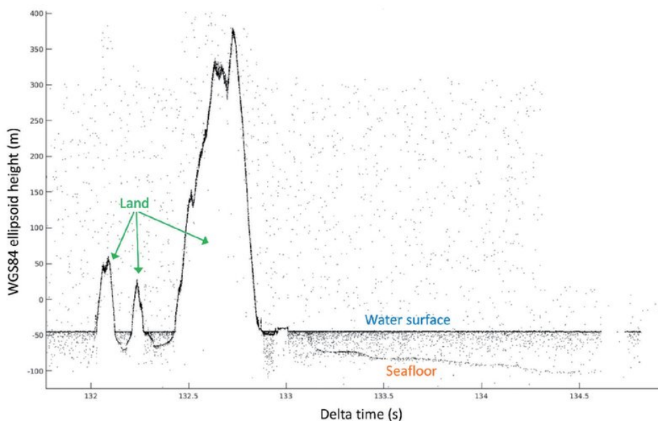
그림 1. ICESat-2의 궤도상 광자 분포와 육상·수면·해저 신호의 구분. 세로축은 WGS84 타원체고 (Parrish et al., 2019).
