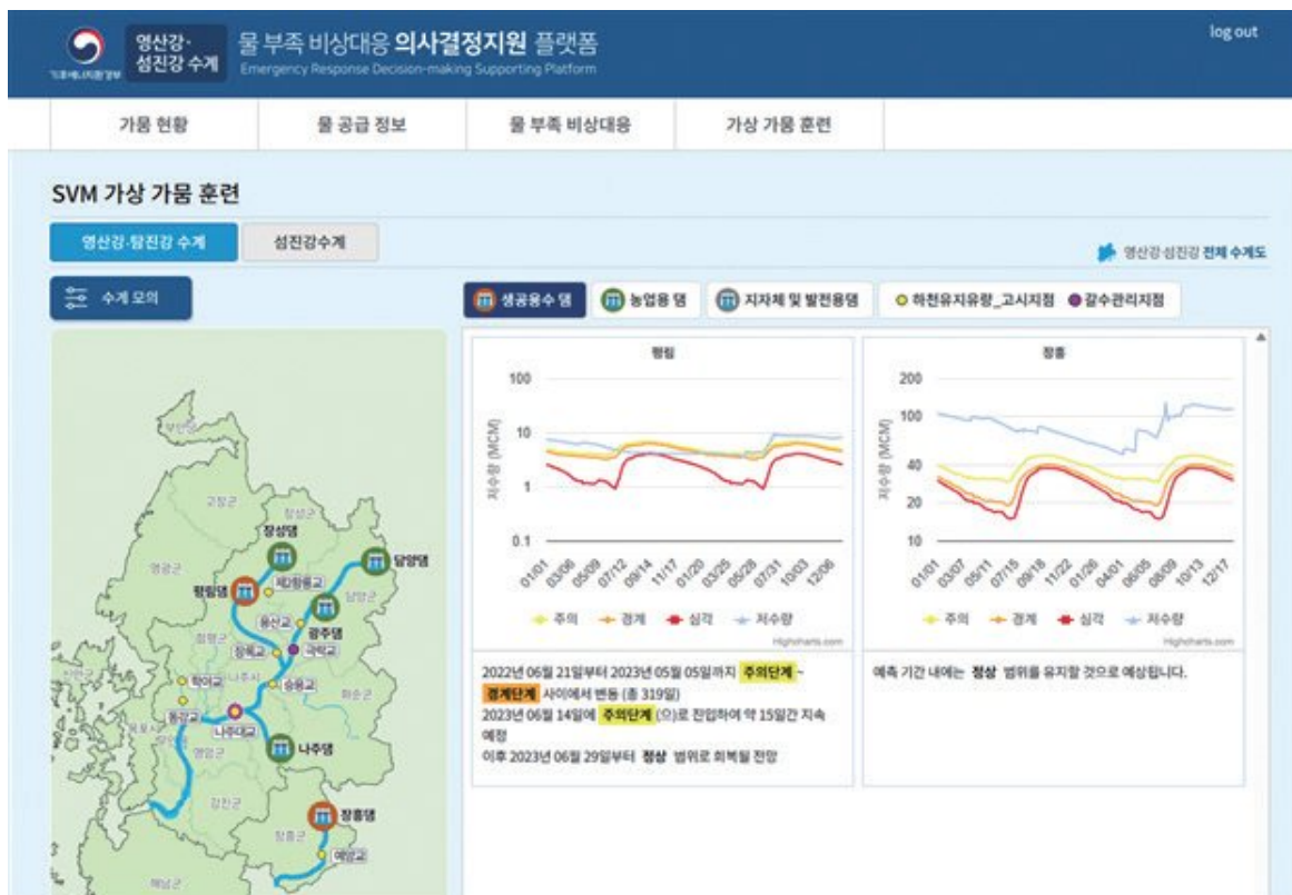
그림 5. 비전공유모형(SVM) 화면
