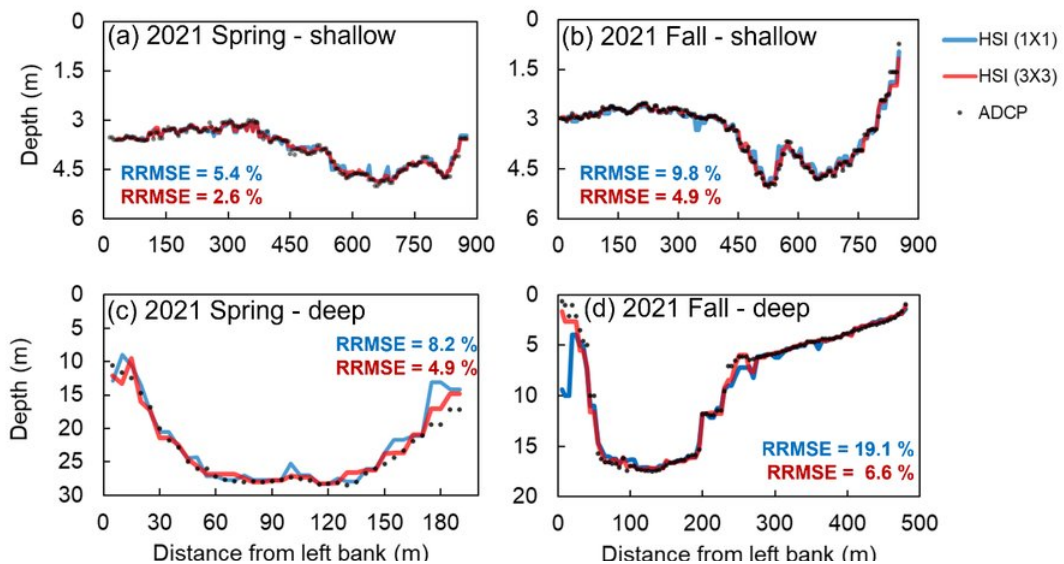
그림 3. Wax Lake Delta의 AVIRIS-NG 추정 수심과 ADCP 관측 수심 비교: (a, b) 봄·가을의 얕은 단면, (c, d) 봄·가을의 깊은 단면. 파란색은 원영상(1×1 화소), 빨간색은 3×3 화소 공간 평균을 적용한 결과이며 검은 점은 ADCP 관측값(Kwon et al., 2024).
