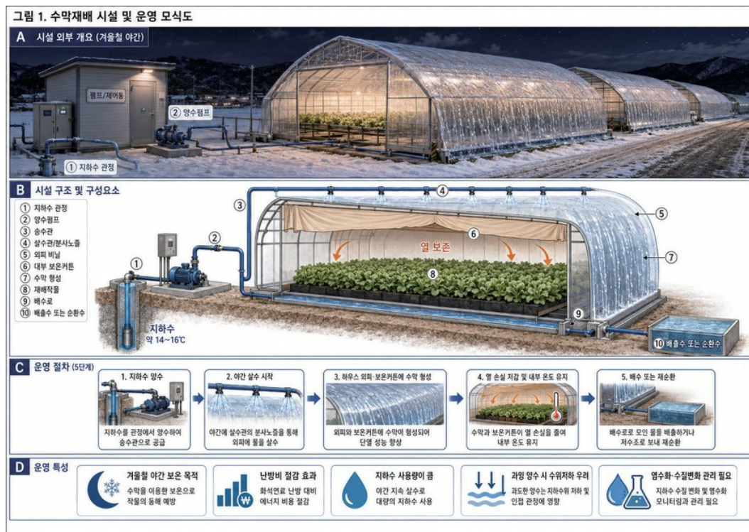
그림 1. 수막재배 시설 및 운영 모식도.
