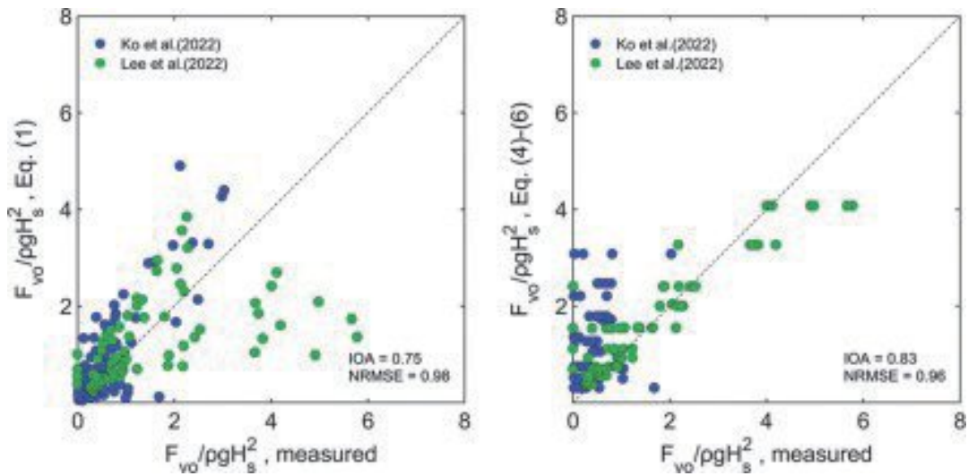
그림 3. 두 실험 자료에 대한 기존 경험식의 적용 결과(좌: Ko et al.(2022)의 식, 우: Lee et al.(2022)의 식)
