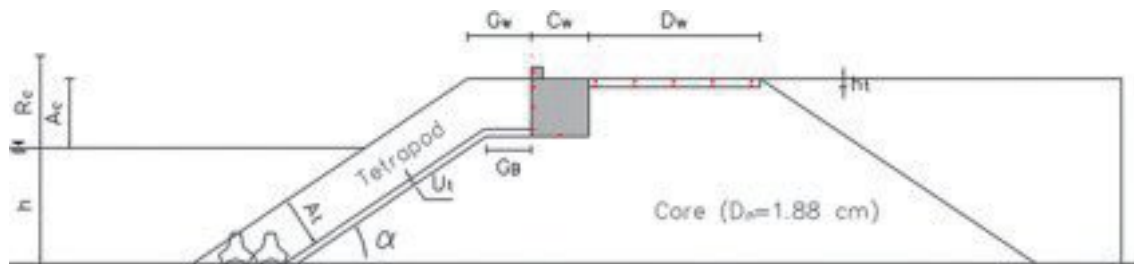
그림 1. Ko et al.(2022)의 실험 단면 및 매개변수 정의
